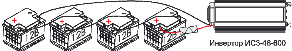
Схема подключения ИС3-48-600.
