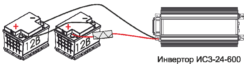
Схема подключения ИС3-24-600.
